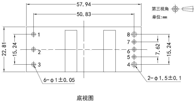
不带散热片
